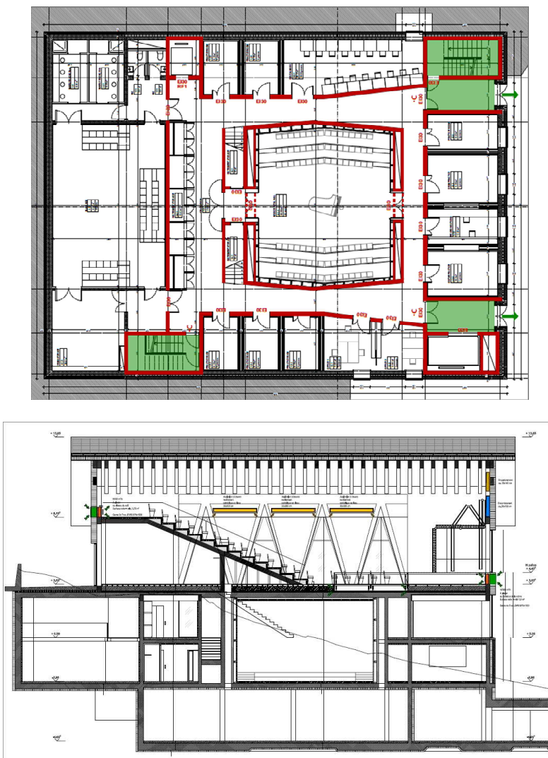
Fig. 1 : Plan des salles de musique et coupe schématique du bâtiment
